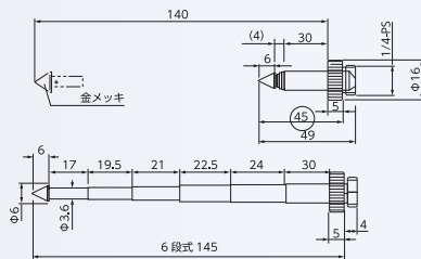
■寸法図 (L100)
