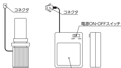
▲本体 (LP-2000-0)
